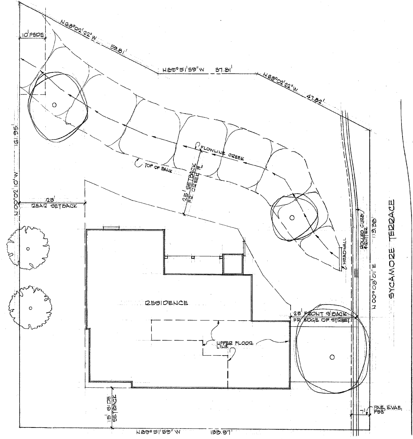
SITE PLAN SCALE: 1" = 10'
